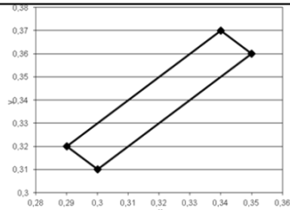
Rysunek 1 - Współrzędne chromatyczności x, y barwy białej
