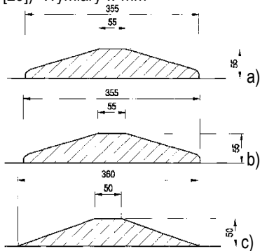
ZAŁĄCZNIK 4 KSZAŁT I WYMIARY W PRZEKROJU POPRZECZNYM PRZYKŁADOWYCH PROGÓW PODRZUTOWYCH (wg [23]) Wymiary w mm
