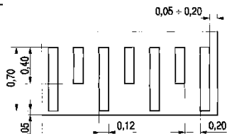
2.2. Przykład oznakowanie listwowego progu zwalniającego (U-16a)
