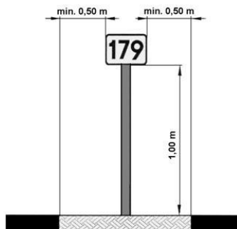
Rys. 3. Słupek krawędziowy U-2
