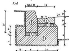
WYMIARY UZUPEŁNIAJĄCE (alternatywne)
