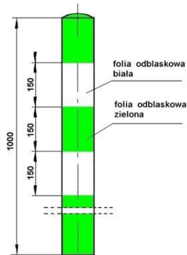
Rys. 3. Słupek krawędziowy U-2
