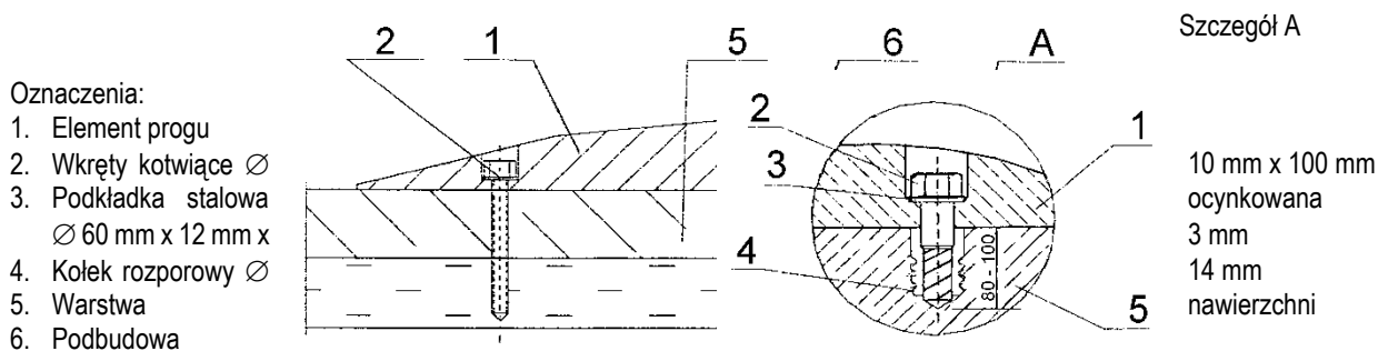
Rys. 4. Przykład umocowania progu do nawierzchni jezdni
