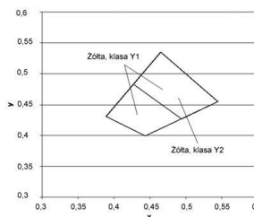
Rys.2. Współrzędne chromatyczności x,y dla barwy żółtej oznakowania
