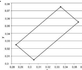
Rys. 1. Współrzędne chromatyczności x,y dla barwy białej oznakowania
