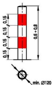
Rys. 5. Słupek blokujący U-12c
